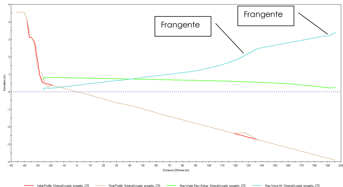
Figura 40 Andamento del profilo d'onda a S'Arena Scoada per mareggiate da 270°N, Tr=50 anni nello stato di progetto
