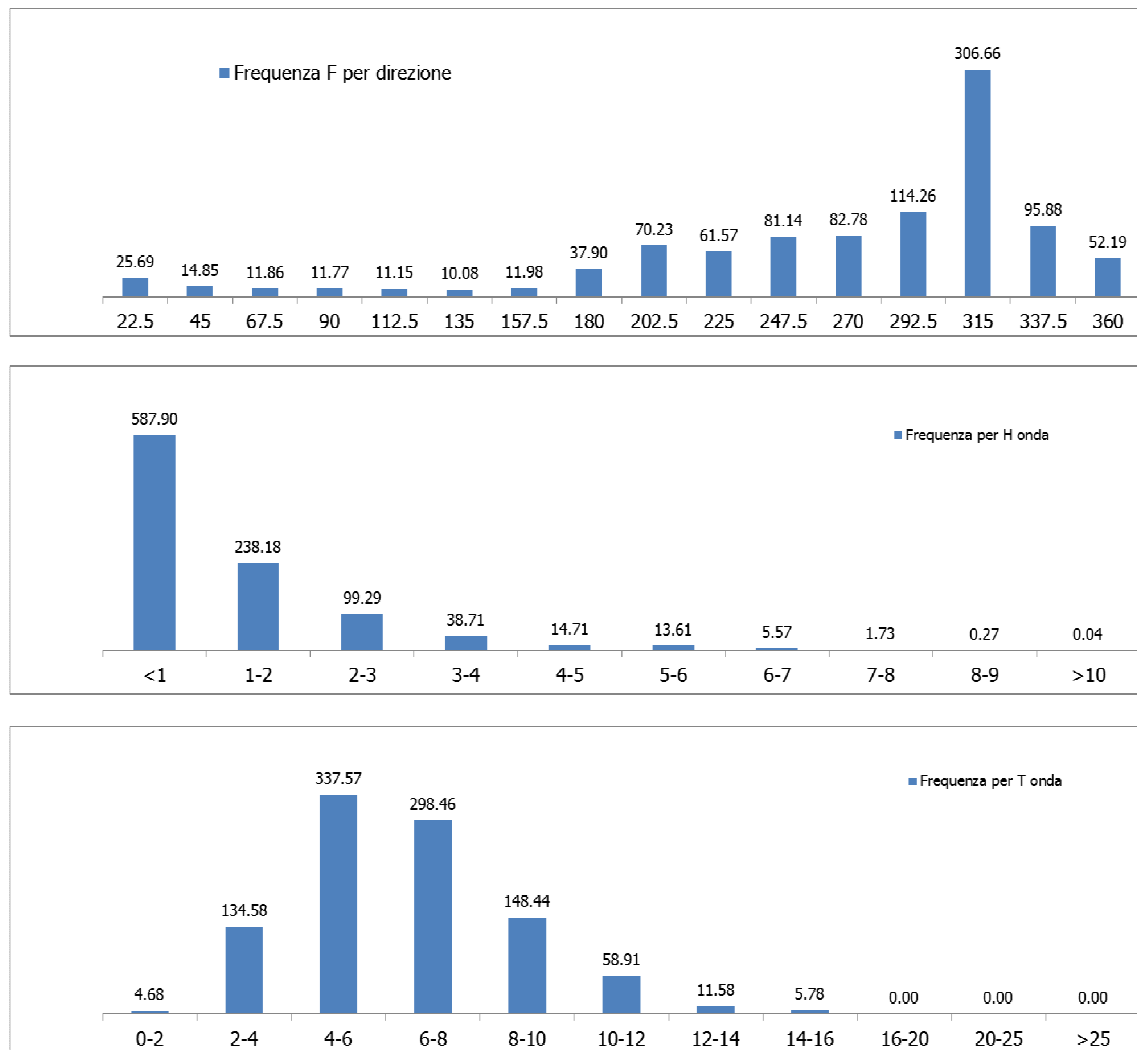
Figura 19- Clima ondoso trasposto al paraggio di Capo Mannu con i dati d'onda trasposti da Alghero
