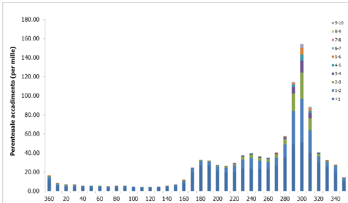
Figura 17- Clima ondoso alla Boa RON di Alghero per direzione e classi di altezza d'onda
