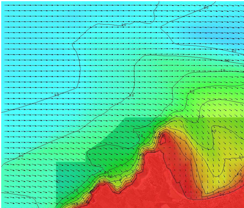
Figura 32 Dettaglio del piano d'onda a Su Pallosu caso 2 (Dir=270°N)
