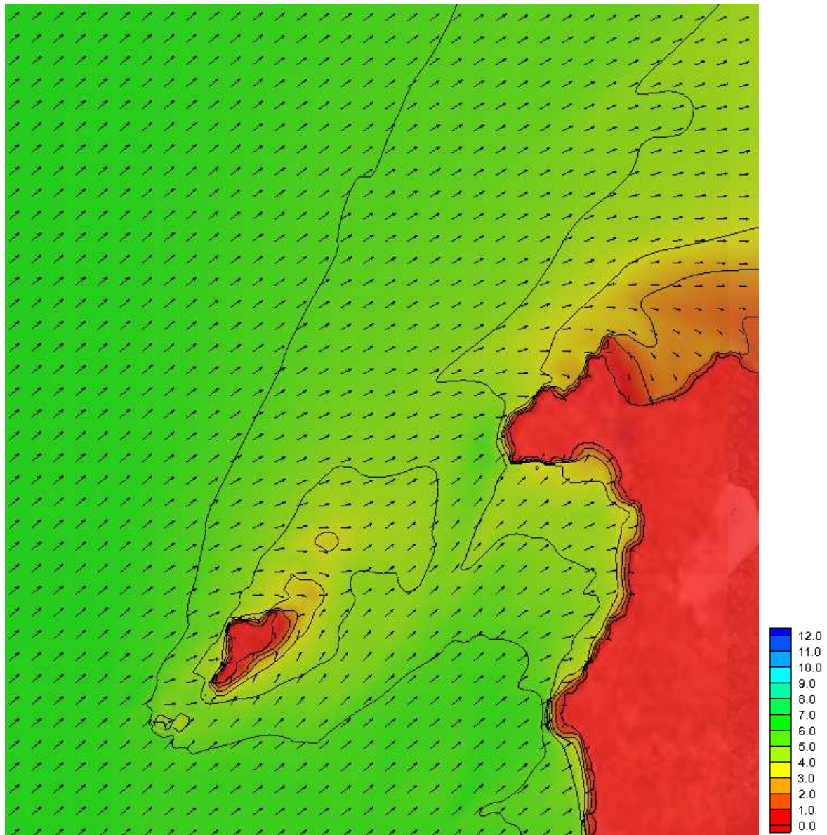
Figura 24 Piano d'onda caso 1 (Dir=225° N)-legenda altezza d'onda in m
