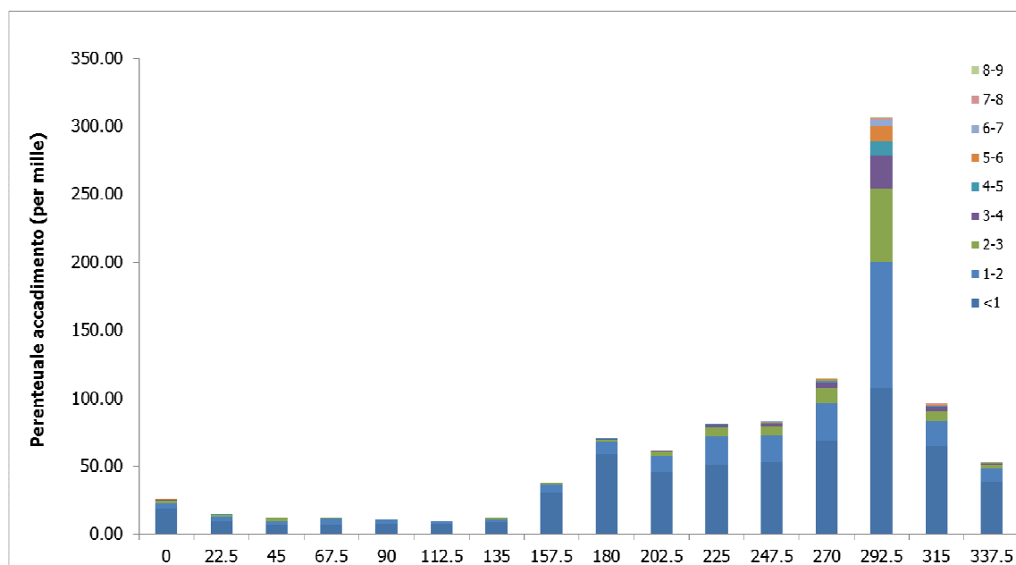
Figura 20- Clima ondoso trasposto al paraggio di Capo Mannu con i dati d'onda trasposti da Alghero
