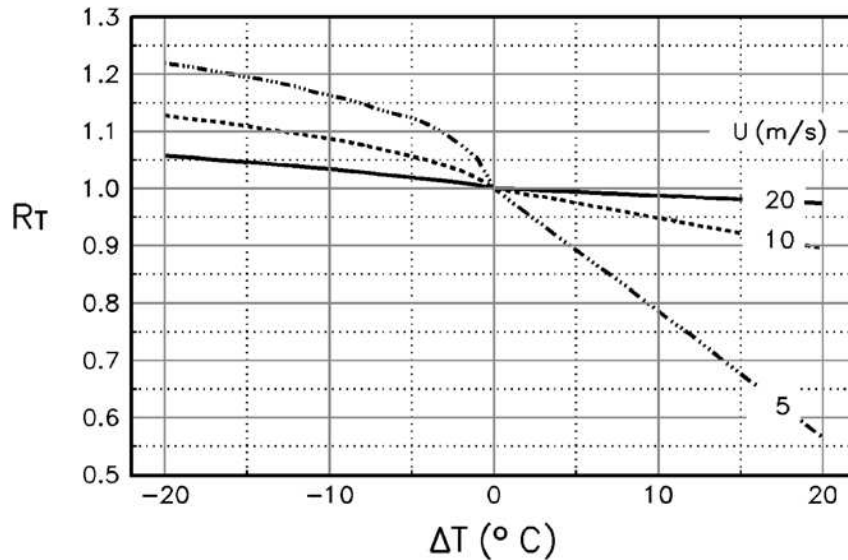
Figura 8 Fattore di correzione in funzione della diversa temperatura aria-mare
