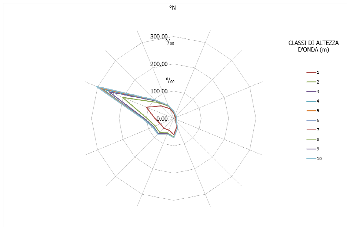
Figura 18- Rosa dei mari a Capo Mannu con i dati d'onda trasposti da Alghero
