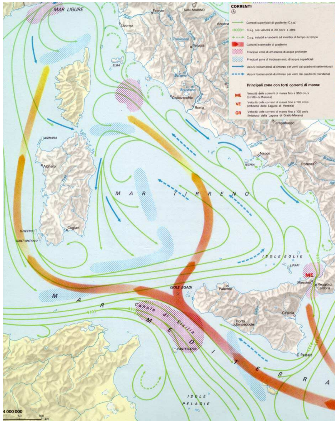
Figura 10 Correnti nel Mediterraneo (da Atlante Tematico CNR)
