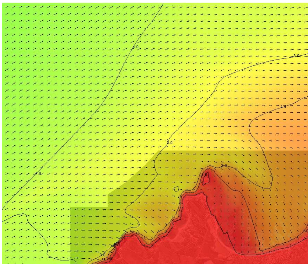
Figura 31 Dettaglio del piano d'onda a Su Pallosu caso 1 (Dir=235°N)
