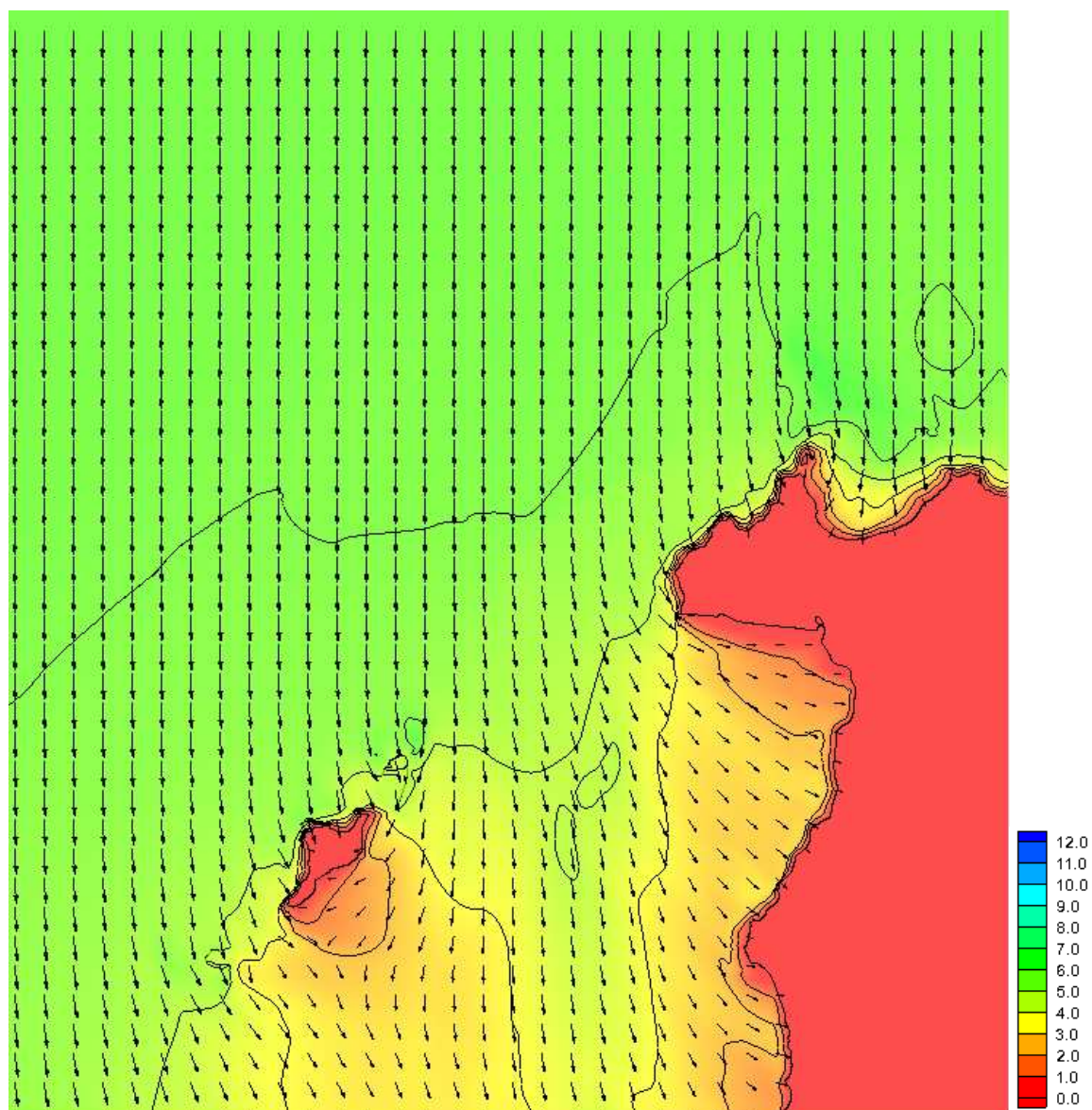
Figura 27 Piano d'onda caso 4 (Dir=0°N)-legenda altezza d'onda in m
