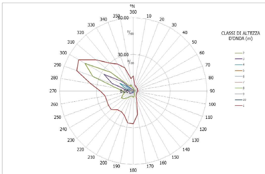
Figura 15- Rosa dei mari alla boa RON di Alghero
