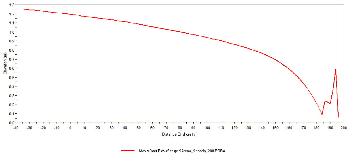
Figura 42 Andamento del sovranzo a S'Arena Scoada per mareggiate come da PGRA, T_r=2 anni
