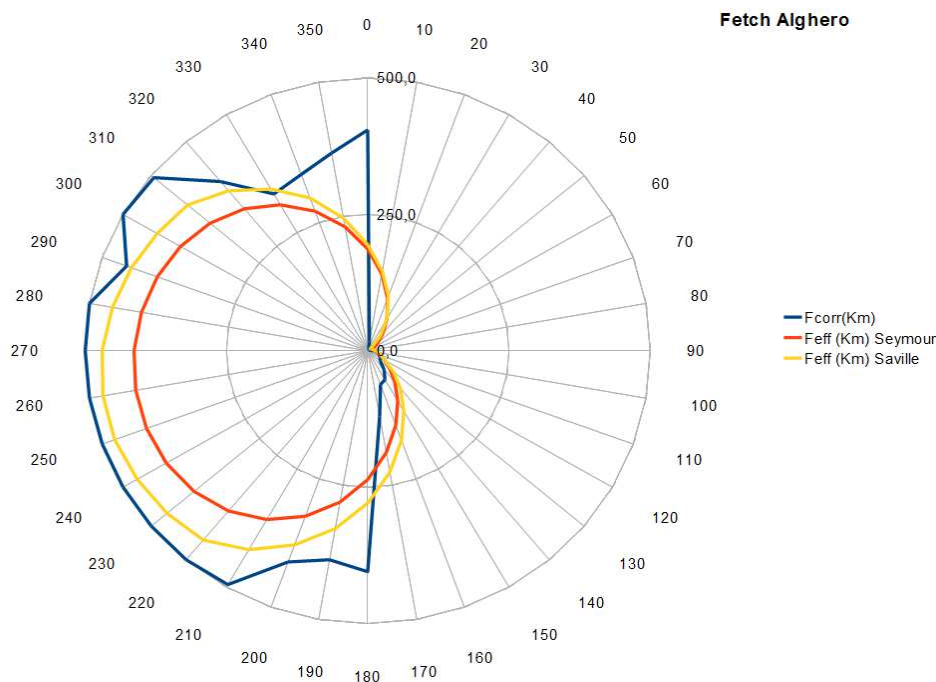
Figura 14 Fetches per il paraggio di Alghero
