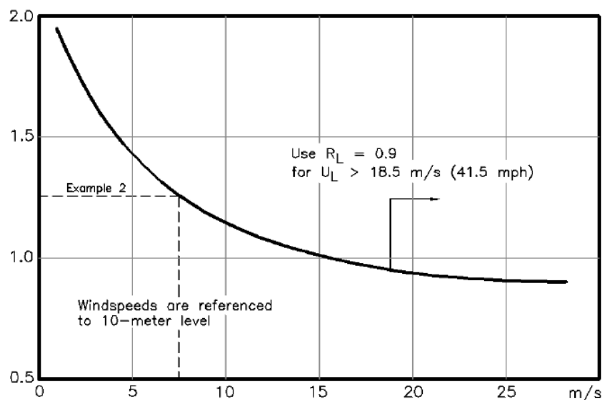
Figura 7 Curva coefficiente R_T in funzione della velocità del vento a terra ( V_T - asse x)- da Coastal Engineering Manual
