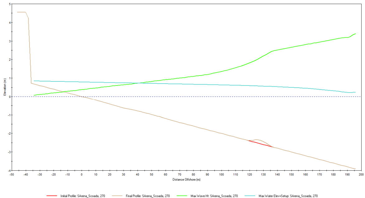
Figura 39 Andamento del profilo d'onda a S'Arena Scoada per mareggiate da 270°N, Tr=50 anni nello stato attuale
