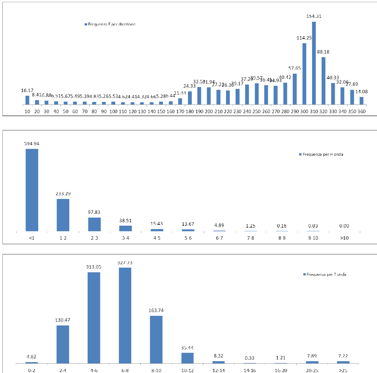
Figura 16- Clima ondoso alla boa Ron di Alghero
