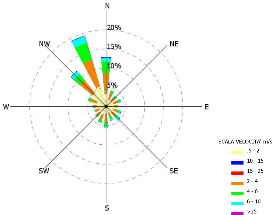
Figura 6 Rosa del regime dei venti per il paraggio di Carloforte (periodo 1998-2009)
