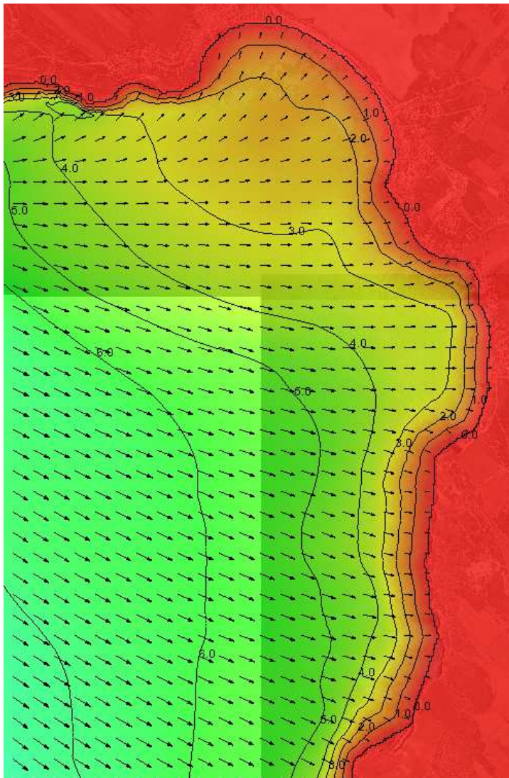
Figura 30 Dettaglio del piano d'onda a S'Arena Scoada caso 3 (Dir=315°N)
