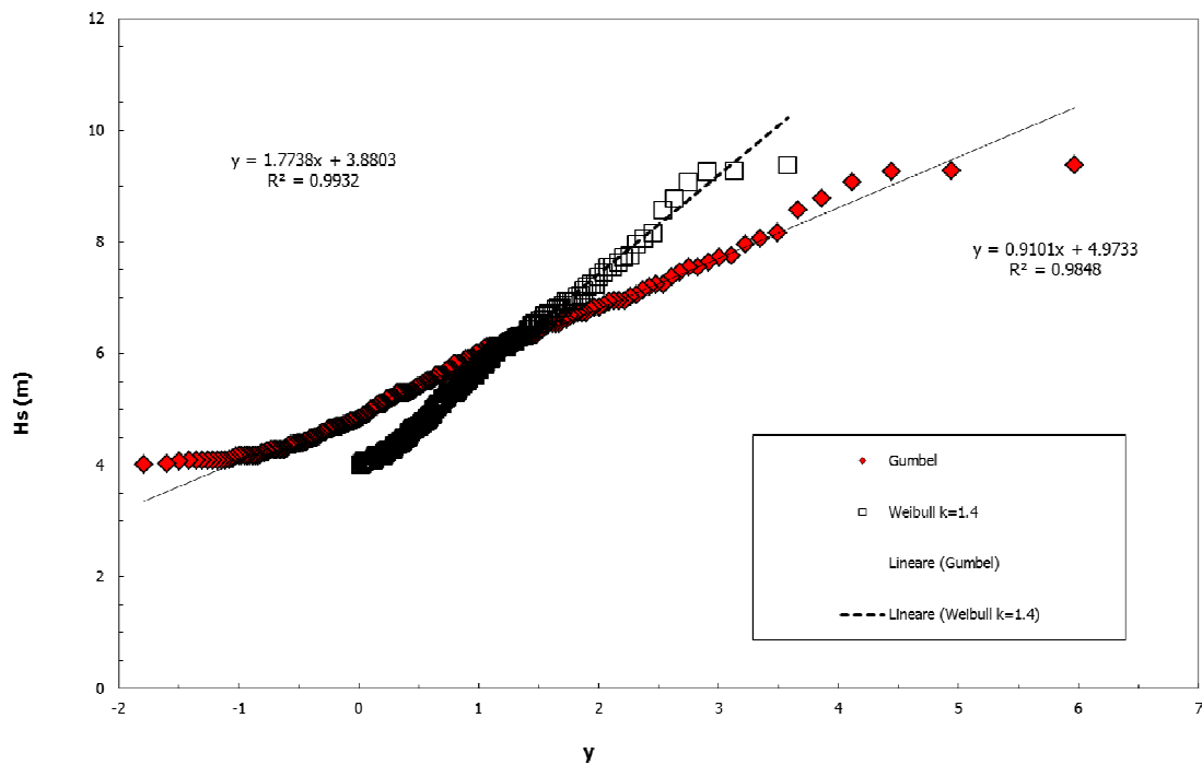
Figura 21 Andamento dei dati sul piano di Gumbel dei dati impiegati per la statistica nel settore 292.5-337.5°N (direzione 315°N)
