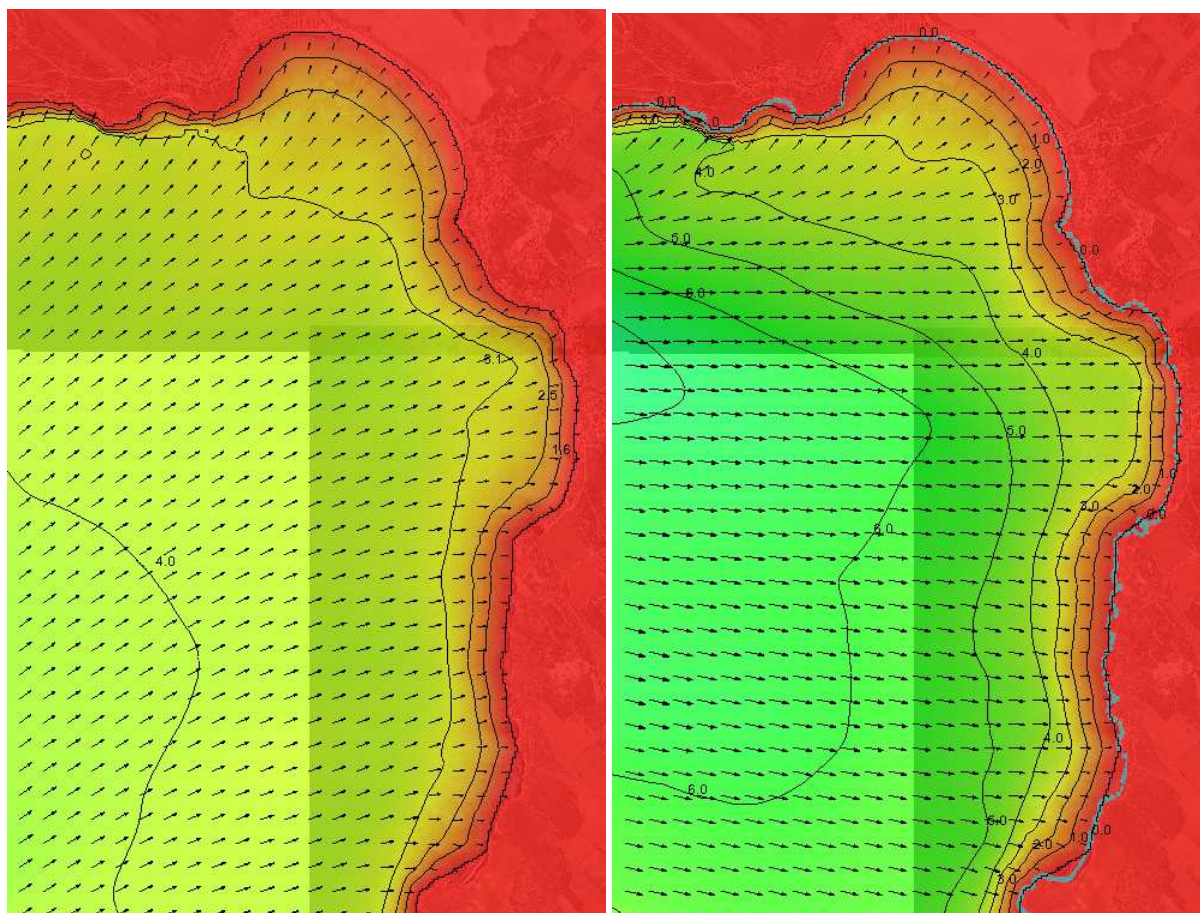
Figura 29 Dettaglio del piano d'onda a S'Arena Scoada caso 1 (Dir=235°N) e caso 2 (Dir=270°N)
