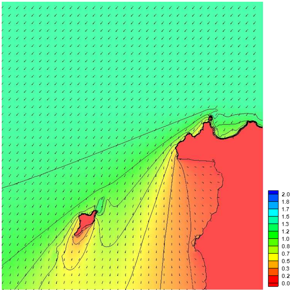
Figura 28 Piano d'onda caso 5 (Dir=45°N)-legenda altezza d'onda in m
