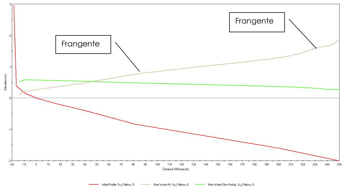
Figura 38 Andamento del profilo d'onda a Su Pallosu per mareggiate da 0°N, Tr=50 anni nello stato attuale
