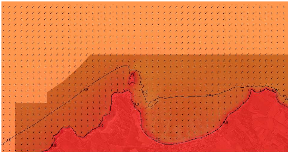
Figura 35 Dettaglio del piano d'onda a Su Pallosu caso 5 (Dir=45°N)
