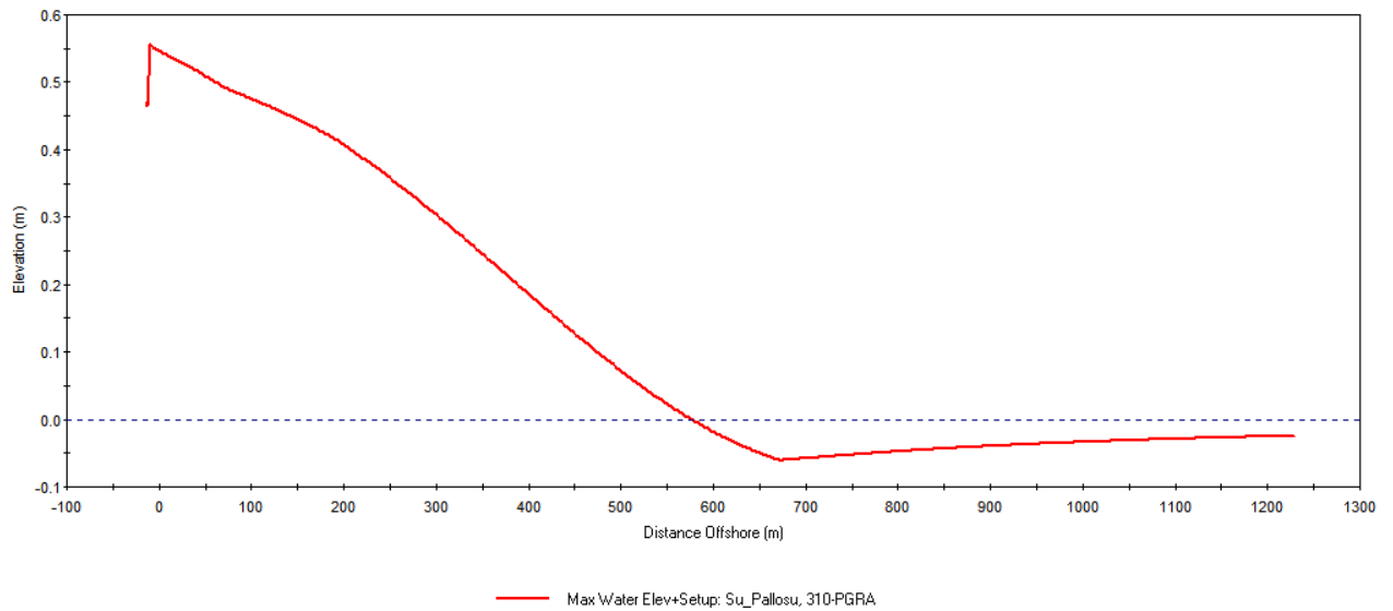
Figura 41 Andamento del sovranzo a Su Pallosu S'Arena Scoada per mareggiate come da PGRA, T_r=2 anni
