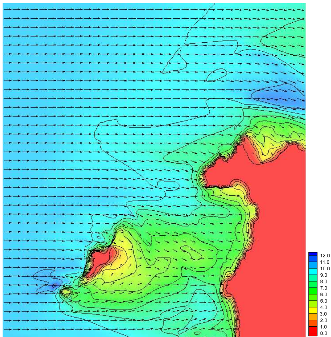
Figura 25 Piano d'onda caso 2 (Dir=270°N)-legenda altezza d'onda in m
