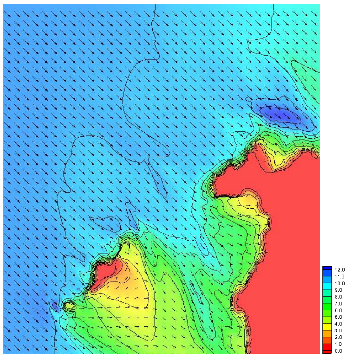
Figura 26 Piano d'onda caso 3 (Dir=270°N)-legenda altezza d'onda in m
